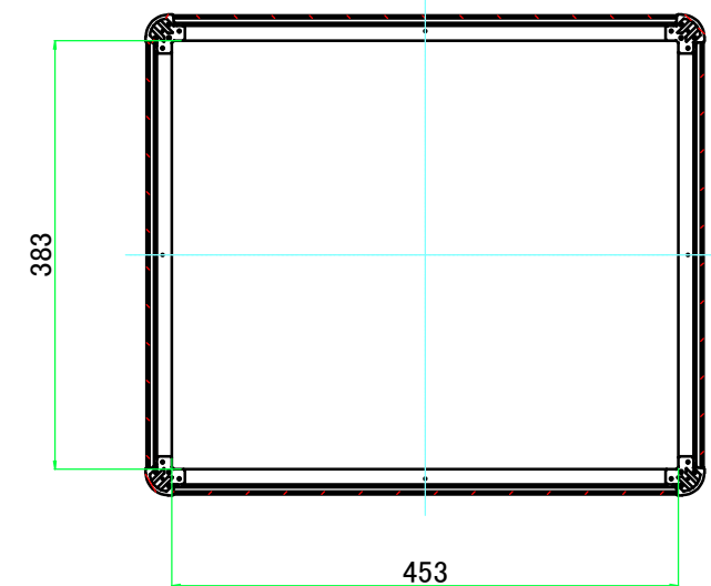
C-C ( 1 : 7.5 )
